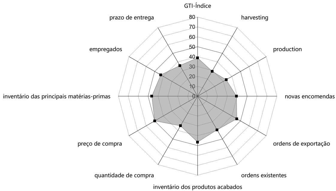
subíndices GTI-Brasil (%)
