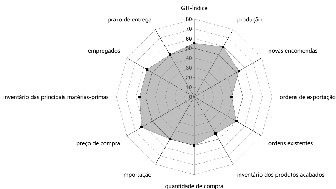
subíndice GTI-China (%)
